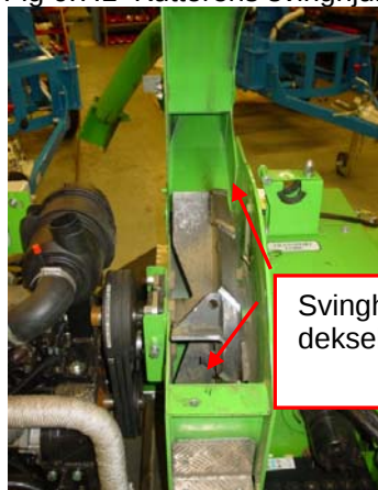
Fig 6.7.1 Kutterens svinghjuldeksel
