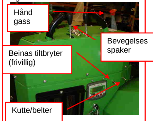
Fig 5.5.1 Beltekontroller
