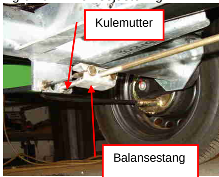
Fig 6.15.2 Bremsejustering
